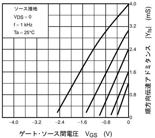
|Yfs| - VGS
