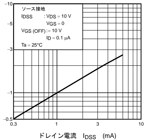
VGS(OFF) - IDSS
