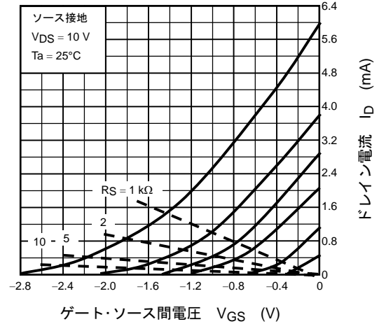
ID - VGS
