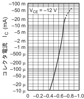
エミッタ接地伝達静特性
