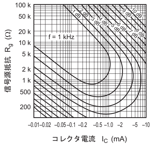
雑音特性 (2)
